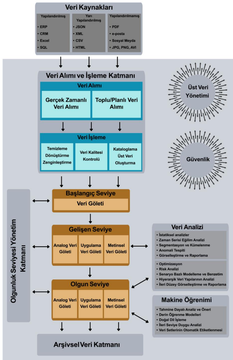
Önerilen Veri Gölü Mimarisi Modeli
